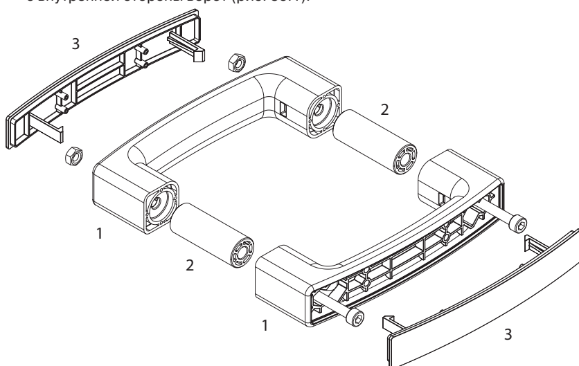
Рис. 36 Комплект ручки HGI006
