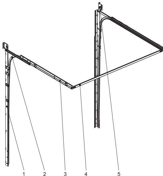
Рис. 10. Схема несущего каркаса ворот.
