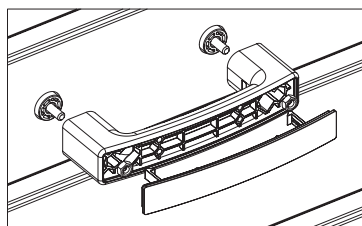
Рис.36.2 Установка ручки. Вид снаружи
