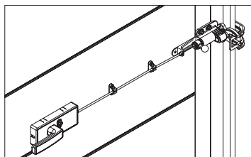
Рис. 40.1. Устройство запирающее Вид изнутри
