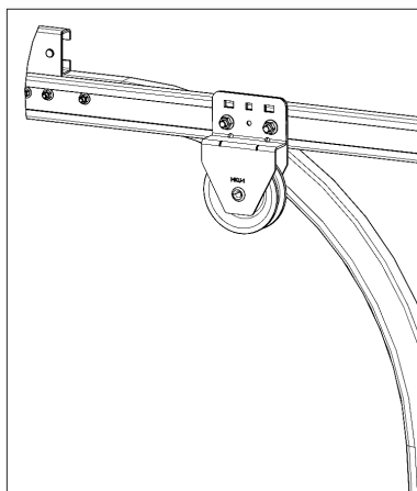
Рис. 41.1. Крепление блока НКU001 к горизонтальной направляющей.
