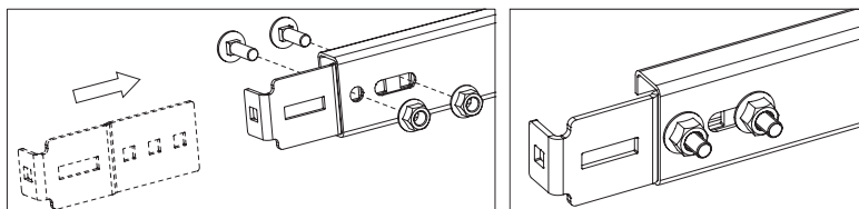
Рис. 6. Сборка мерной планки.
