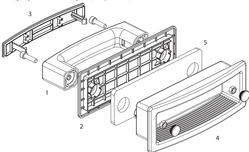
Рис. 37 Комплект ручки НГИ007
