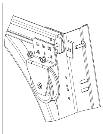
Рис. 41.1. Крепление блока НКU001 к горизонтальной направляющей.
