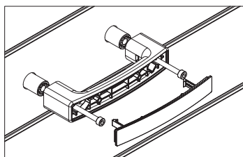
Рис.36.1 Установка ручки. Вид изнутри
