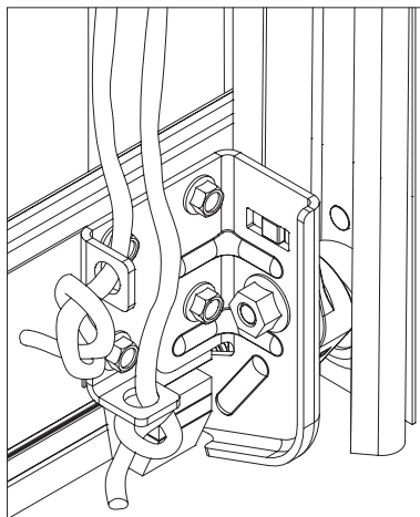
Рис. 41.2. Крепление каната.
