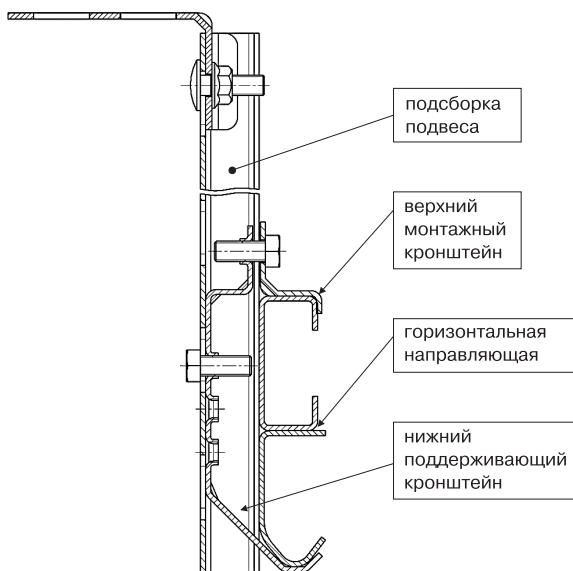
Рис. 20.2. Сборка подвеса.
