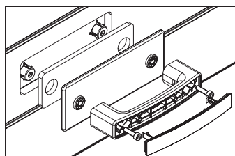
Рис.37.2 Установка ручки. Вид изнутри
